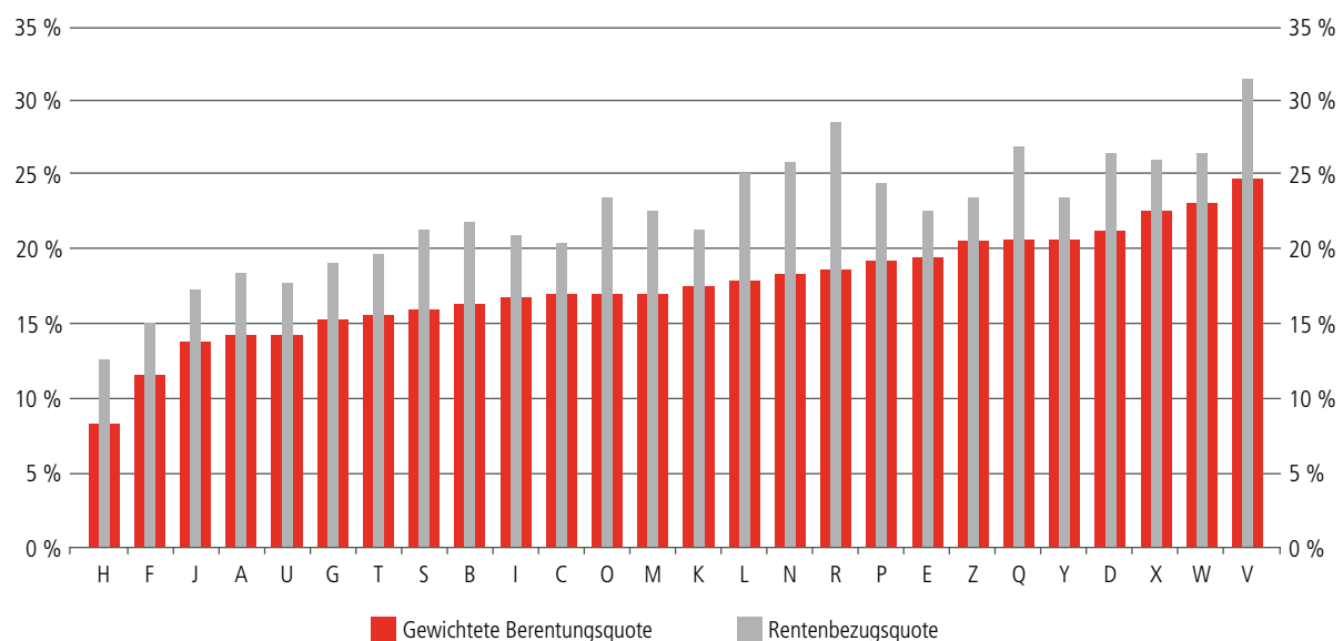
Gewichtete Berentungsquoten in aufsteigender Reihenfolge und Rentenbezugsquoten (Kohorte Neuanmeldungen 2009 nach IV-Stelle, Stand Ende 2013)
